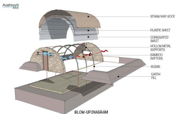
Behelfsunterkunft vom Typ Ashraya
